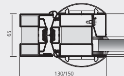
Finger protection door EI30
