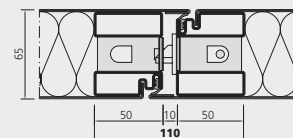
Finger protection door EI30
