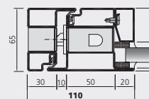
Sheet metal door EI30/EI60
